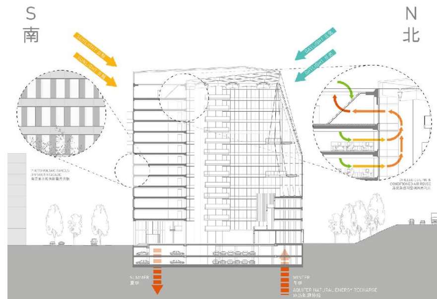
图 4：地下含水层储能技术原理图
