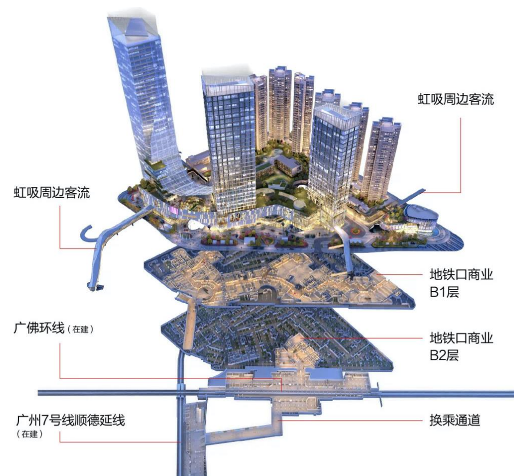
图 1：TOD 项目示意图
