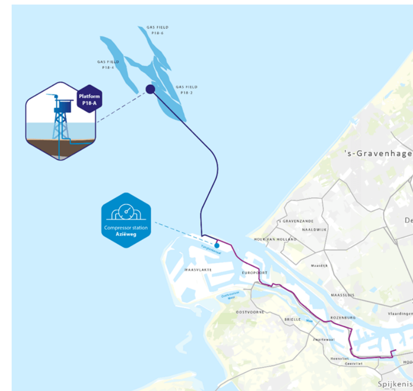
图 14：Porthos 项目的二氧化碳运输和封存路线
