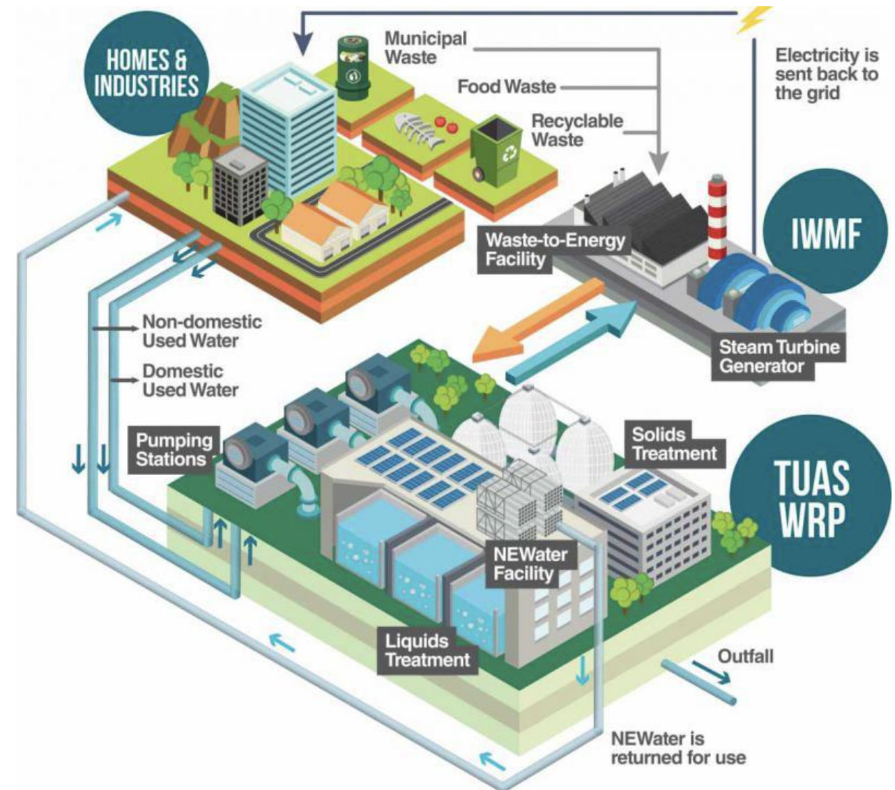
图 16：集污水处理和固废处理于一体的工厂——Tuas Nexus
