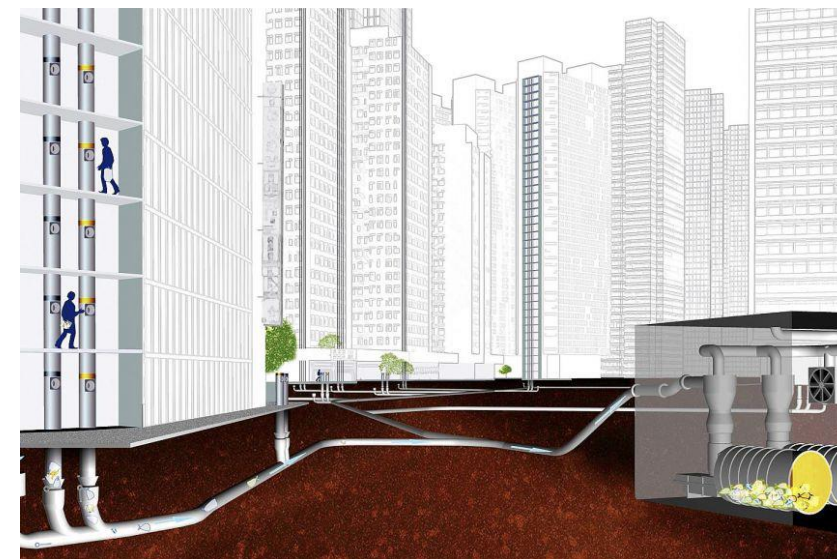
图 15：气动废物输送系统示意图
