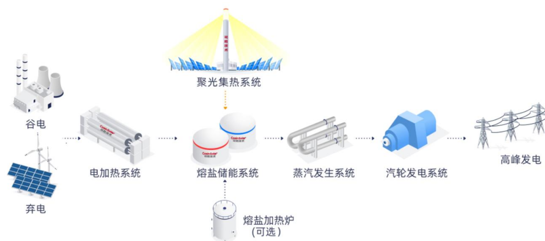
图 20：光热型熔盐储能电站流程图
