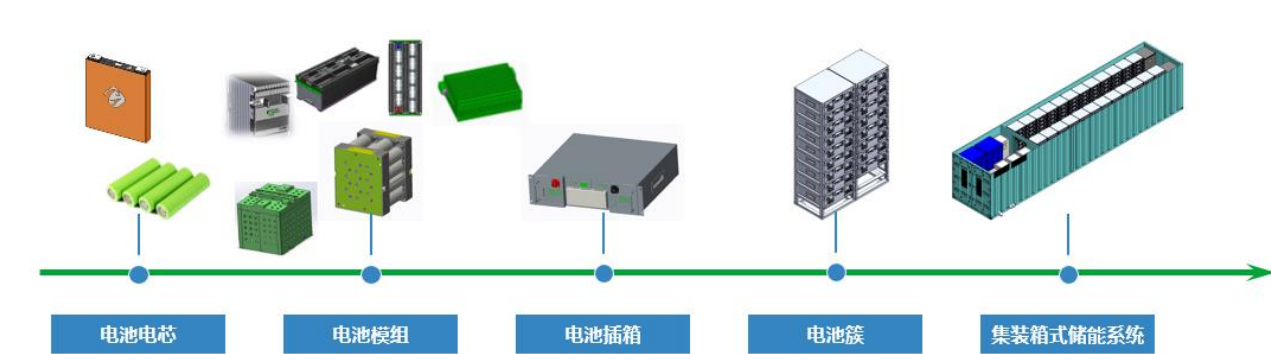
图 9：电池组结构简图
